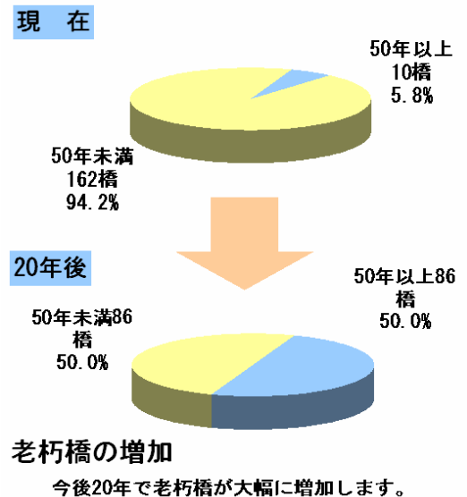
図 1.1 老朽化橋の増加
