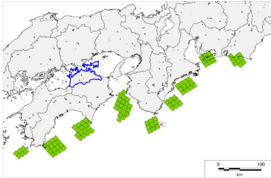
①1707年 宝永地震 (M8.6)
