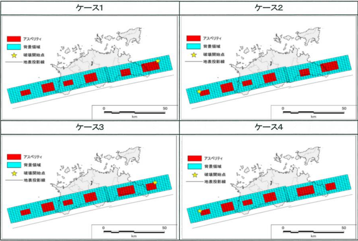
【中央構造線（断層モデル）】
