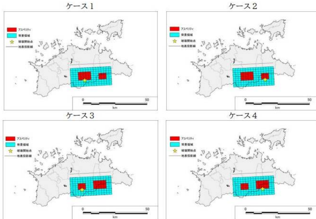
【長尾断層（断層モデル）】
