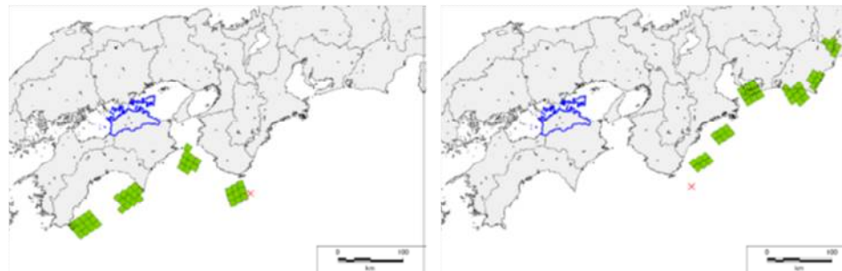
②1854年 安政南海地震 (M8.4) ②1854年 安政東海地震 (M8.4)
